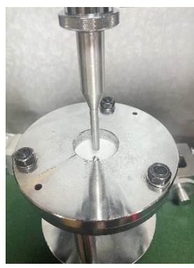
貫通抵抗力試験
